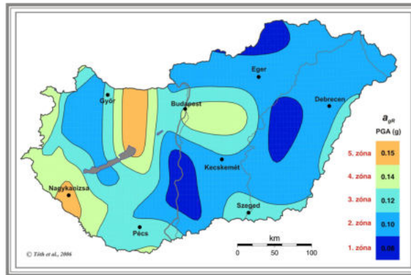
Magyarország szeizmikus zónatérképe [Földrengések következtében 50 év alatt, 10%-os meghaladási valószínűséggel, az alapkőzeten várható vízszintes gyorsulás g (gravitációs gyorsulás) egységben. (forrás: foldrenges.hu)
