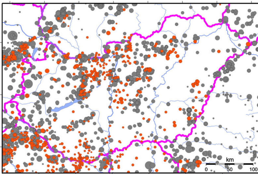
A földrengések területi eloszlása Magyarországon. A szürke körök a historikus rengéseket (1456-1994), a piros körök az utóbbi évek rengéseit (1995-2009) mutatják. (forrás: foldrenges.hu)
